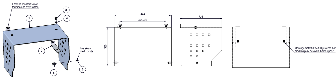
1. Väderskydd | 2. Konsol | 3. Sexkantskruv | 4. Bricka | 5. Gummidämpare | 6. Förs. krysskruv
